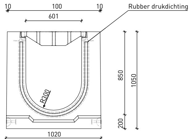
vooraanzicht
